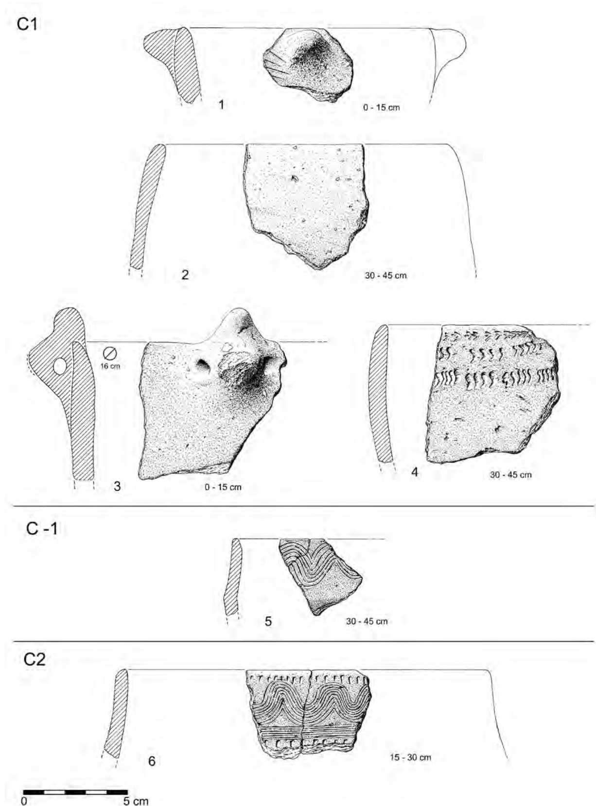
Fig. 18 – Cerâmica (materiais provenientes da escavação dos quadrados indicados). Desenhos de Filipe Martins.
