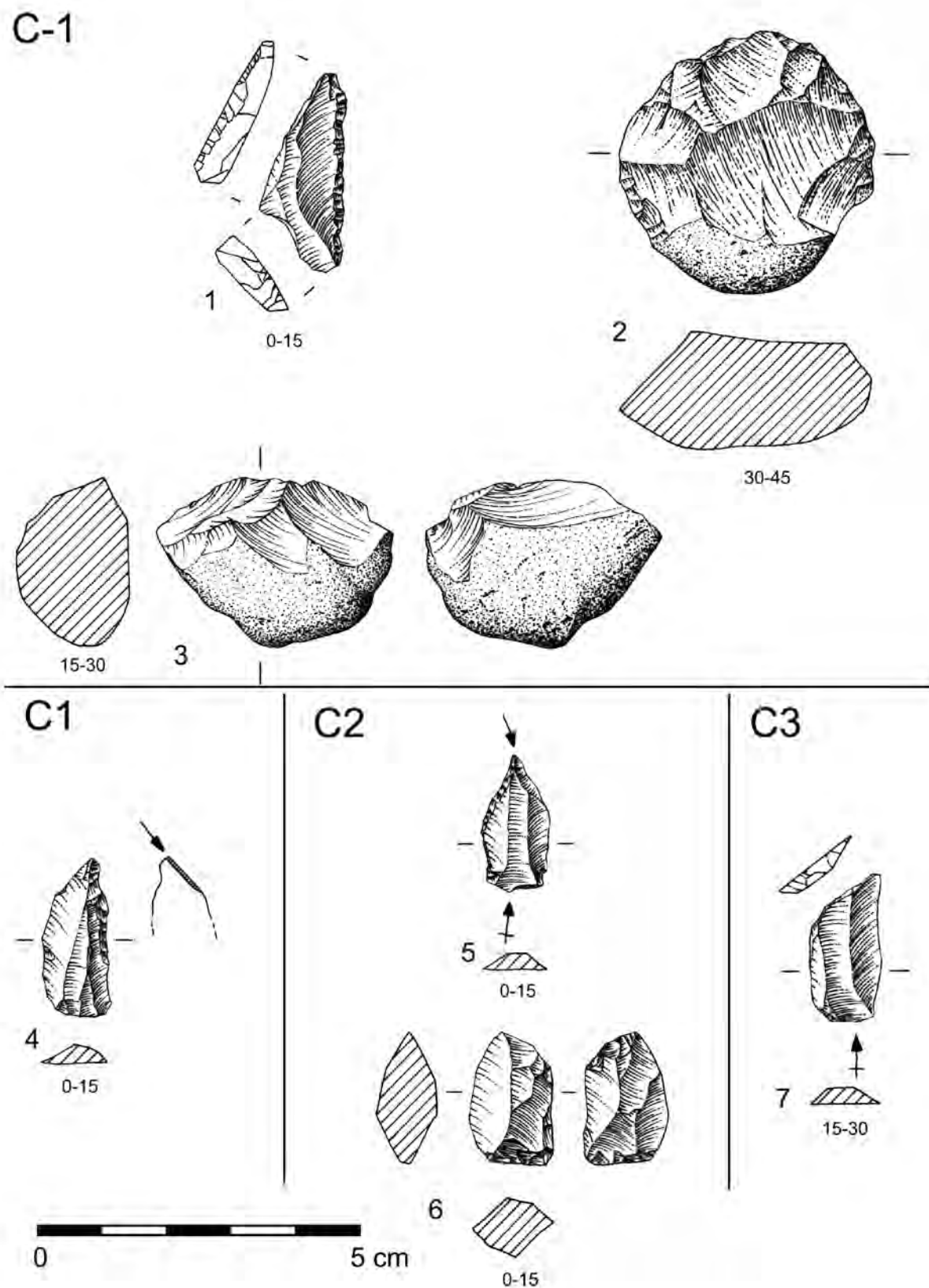
Fig. 9 – Pedra lascada em sílex (materiais provenientes da escavação dos quadrados indicados). Desenhos de Filipe Martins.
