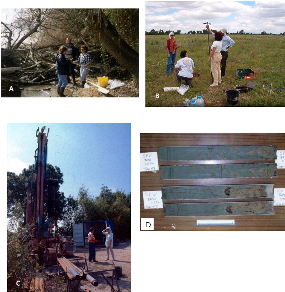
Figura 7. Amostragens manuais: A – Quinta da Boavista; B – Goucharia; amostragem mecânica C- amostragem SEV, amostradores Shelby de 75mm de diâmetro e 1m de comprimento acionados por pressão hidráulica e executados dentro de um furo de sondagem revestido; D-exemplos das carotes. Fotos de Nunes e Azevêdo (em 1999 e 2002).
