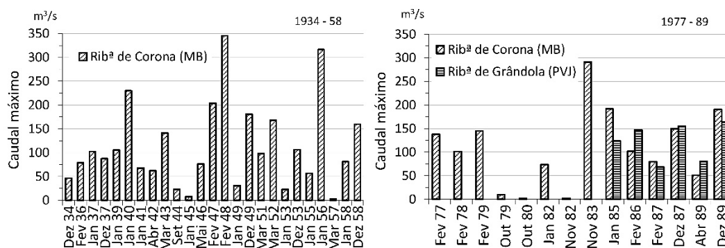
Figura 4. Caudais máximos instantâneos anuais na ribeira de Corona em Moinho do Bravo (MB) nos períodos 1934/35 – 1958/59 e 1976/77 – 1989/90, e na ribeira de Grândola em Ponte Vale Joana (PVJ) no período 1983/84 – 1989/90.
