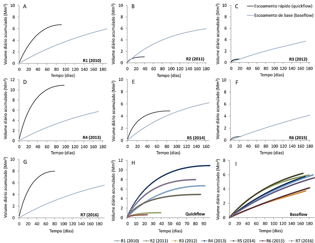
Figura 7. Volume diário acumulado, em Mm 3 , de escoamento rápido e escoamento de base, ao longo de cada recessão (imagens A a G). Volume diário acumulado, em Mm 3 , de escoamento rápido (H) e de escoamento de base (I).
