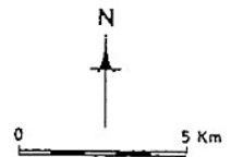
Figura 1. Esboço litológico e tectónico da região onde se insere a área de estudo (adaptado de Cunha, 1989).
