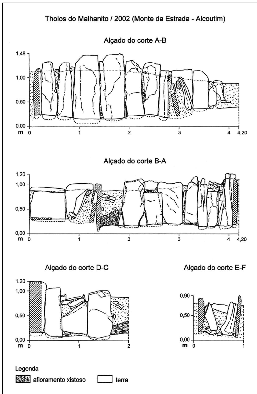
FIGURA 6. Tholos do Cerro do Malhanito. Alçados (ver Fig. 3).
