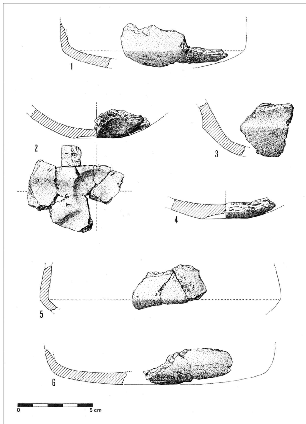
FIGURA 15. Tholos do Cerro do Malhanito. Recipientes do Bronze Final / inícios da Idade do Ferro.
