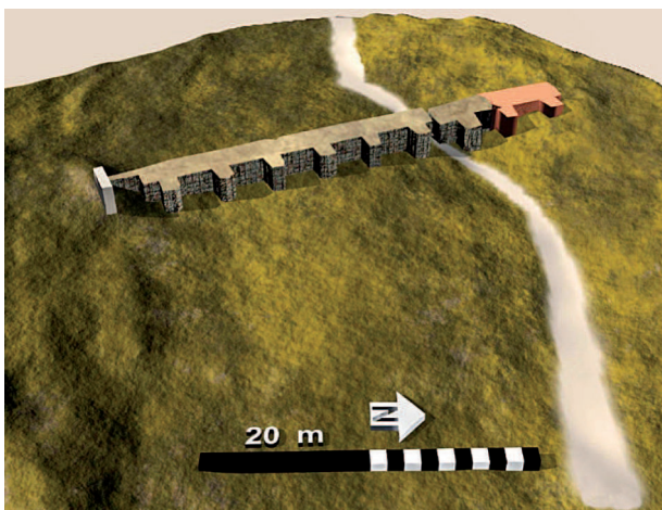
Reconstituição 3D da barragem, vista de jusante
