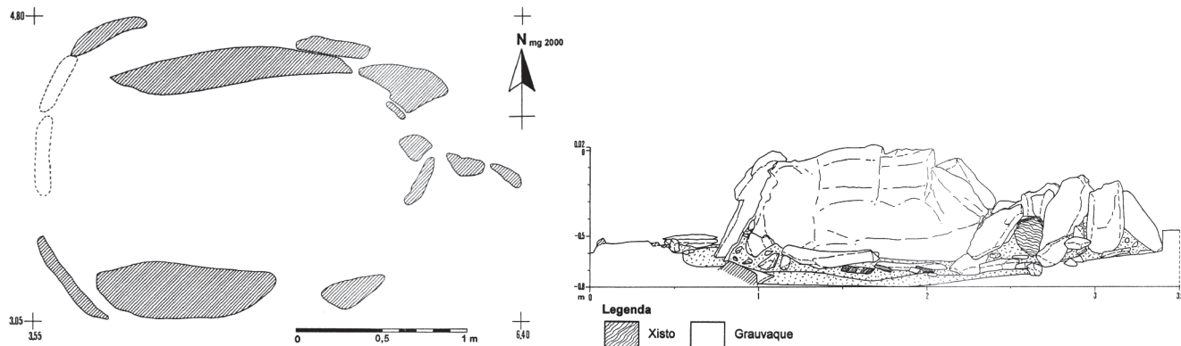
Planta da estrutura e respetivo alçado
