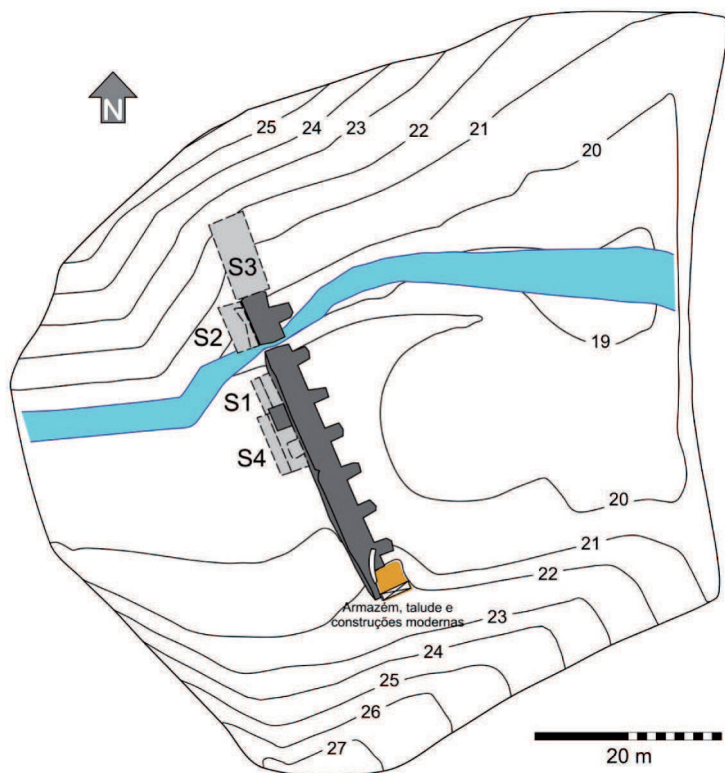
Planta geral da barragem com localização das áreas intervencionadas em 2006/2007
