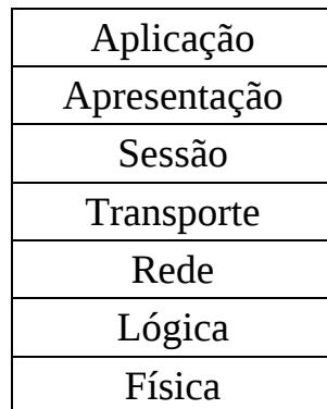
Figura 2 - Modelo OSI
