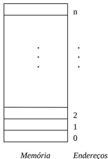
Figura 3 - A memória
