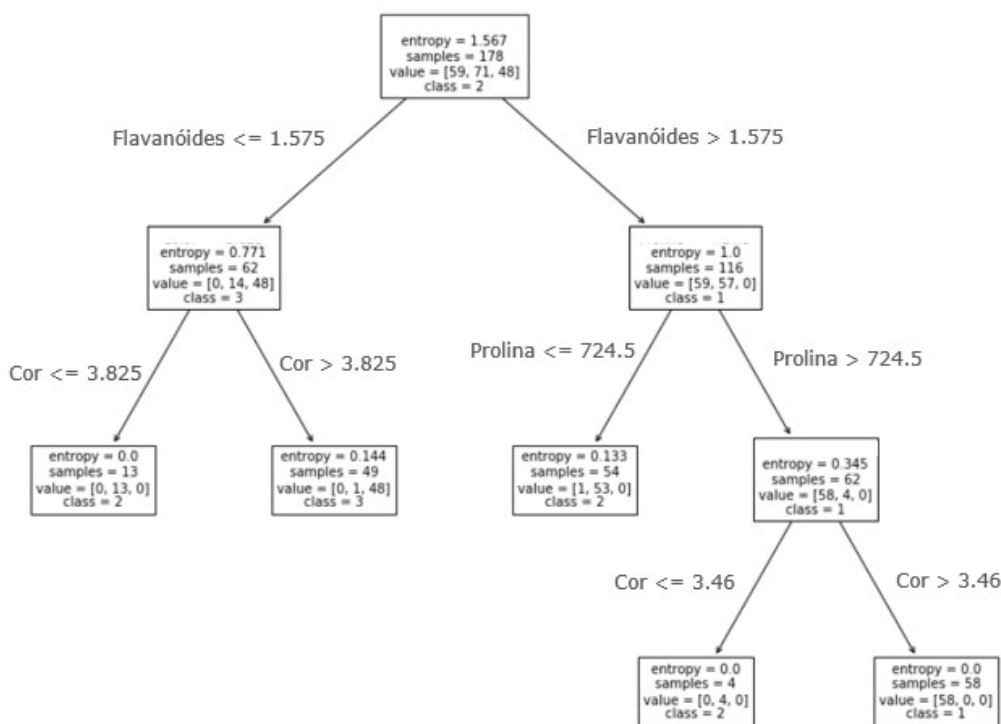
Figura 5. Representação gráfica da árvore de decisão obtida com o dataset “Wine”.
