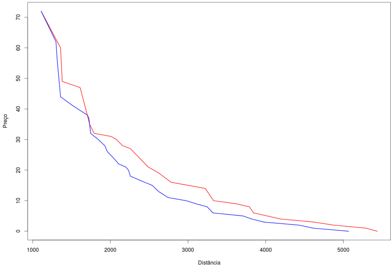
Figura 7.1: Comparação entre os dois algoritmos aproximados para a instância “Singh33_2.33.500.1.5”
