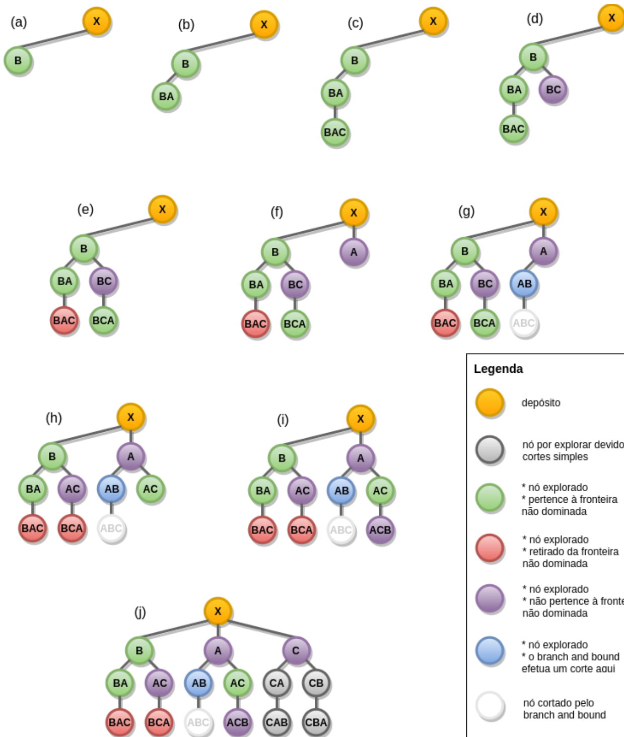
Figura 5.2: Aplicação do algoritmo exato no exemplo ilustrativo
