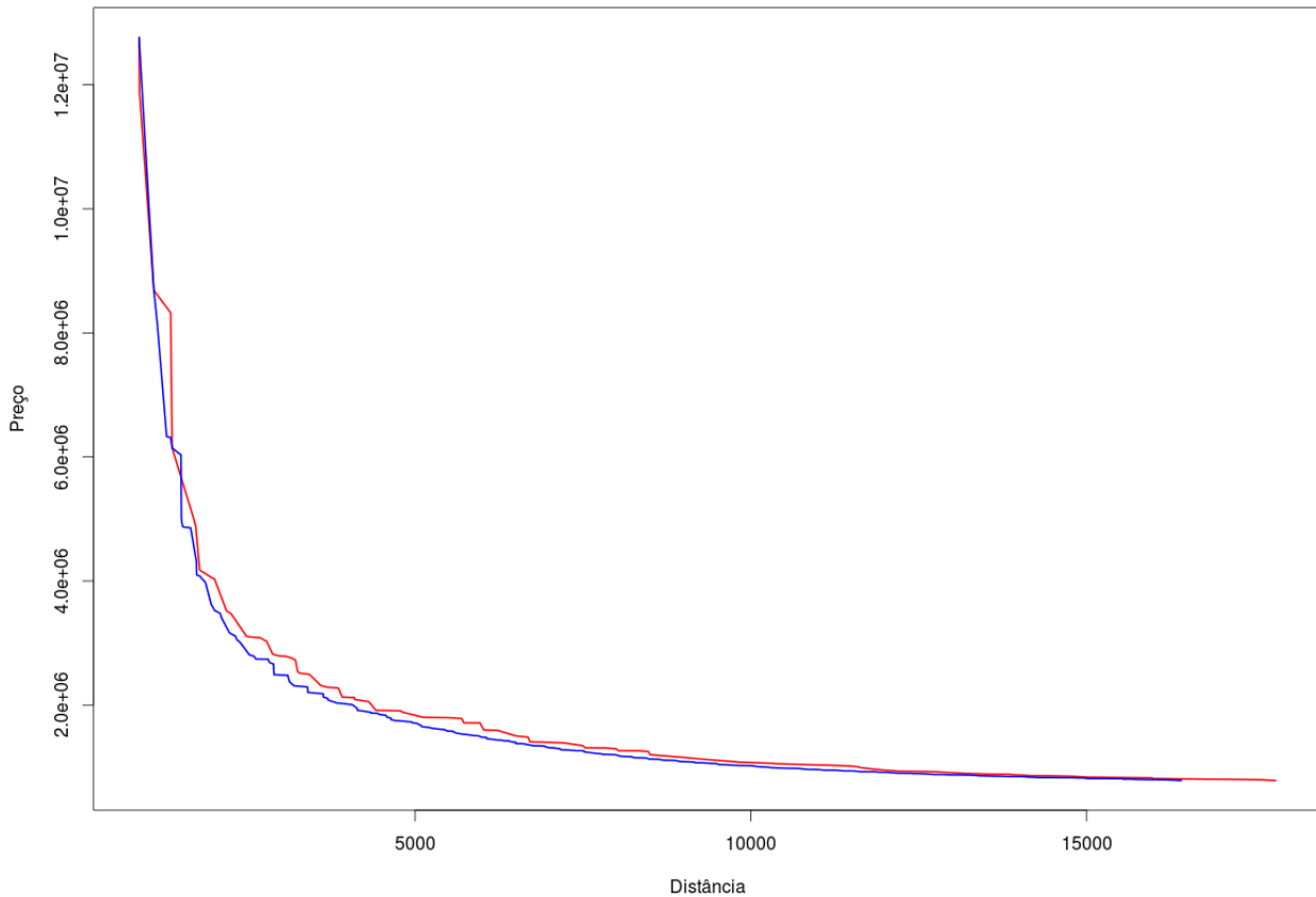
Figura 7.2: Comparação entre os dois algoritmos aproximados para a instância “Singh33_2.33.500.5.50000”
