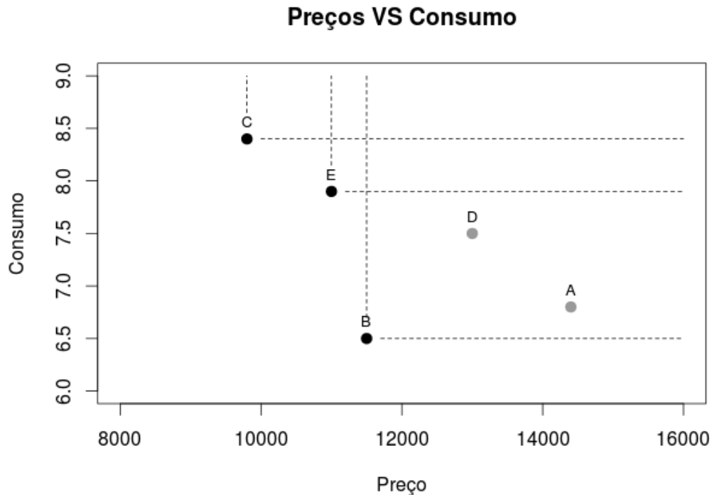
Figura 2.1: Gráfico de preços e consumos em diferentes marcas de carros
