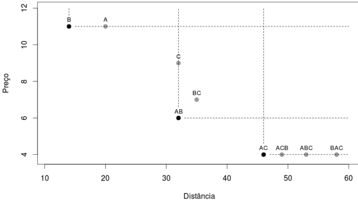
Figura 3.2: Representação gráfica das soluções do exemplo ilustrativo
