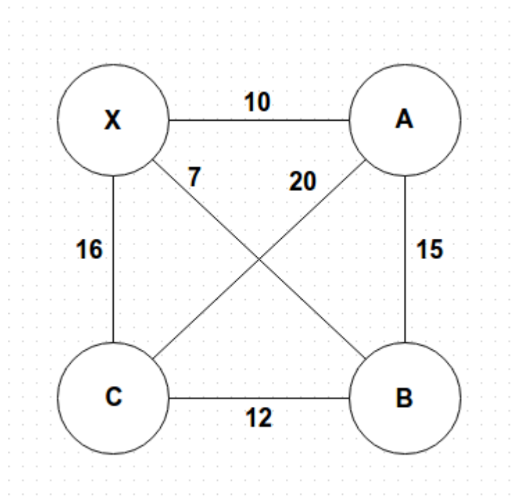
Figura 3.1: Distâncias entre os mercados e depósito do exemplo ilustrativo
