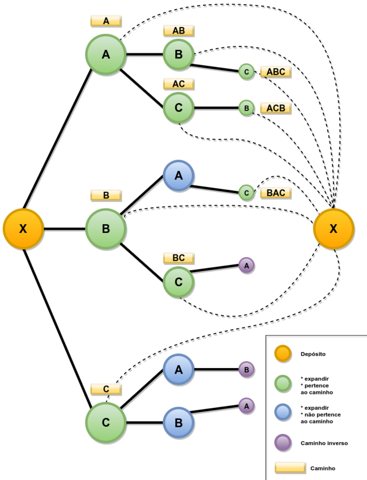
Figura 5.1: Expansão em árvore do exemplo ilustrativo
