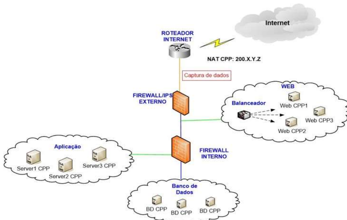
Figura 2. Topologia de rede do CPP
