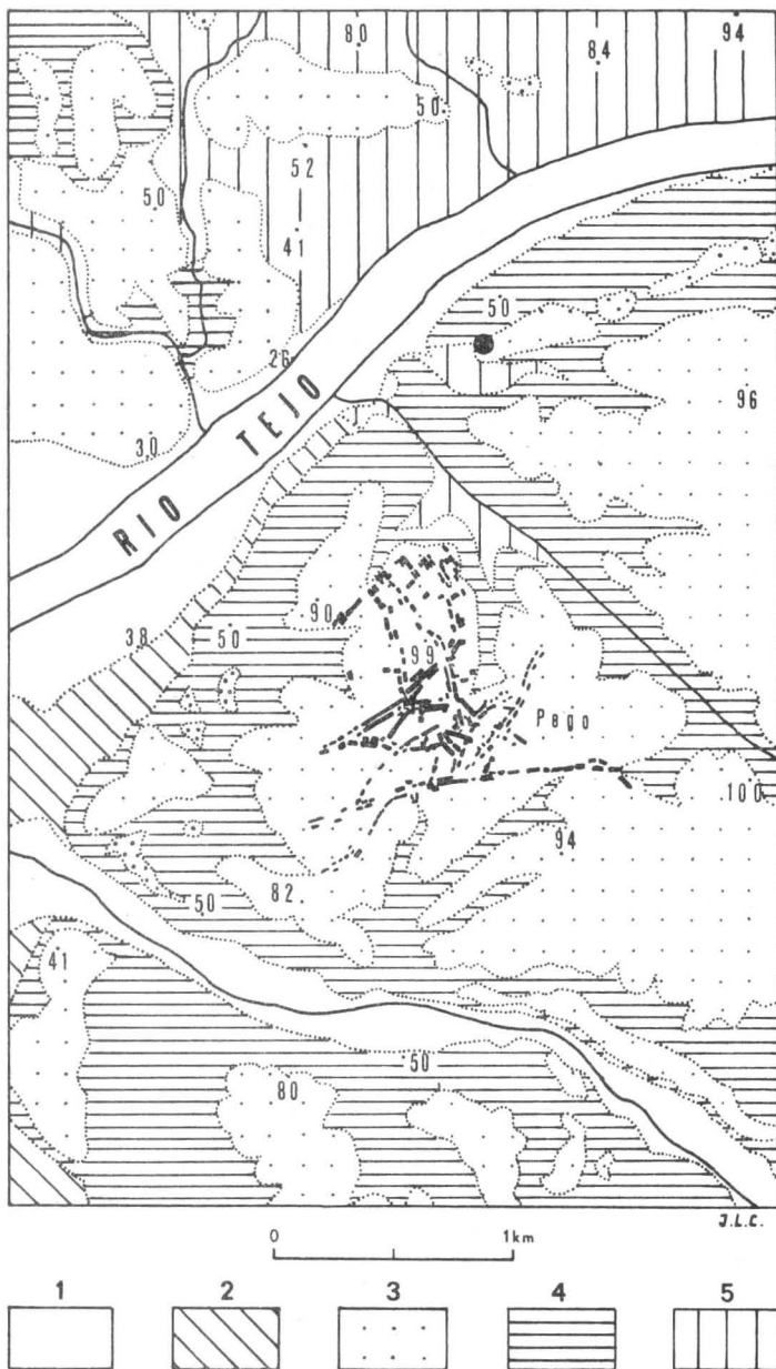
Fig. 1 — Esboço geológico provisório e simplificado da região do Pego, a E de Abrantes.
