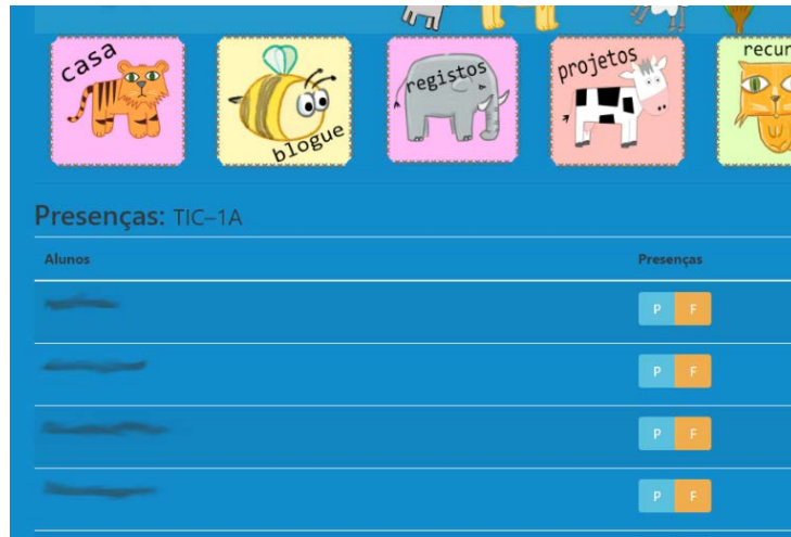
Figura 3.14. Marcar Presenças
