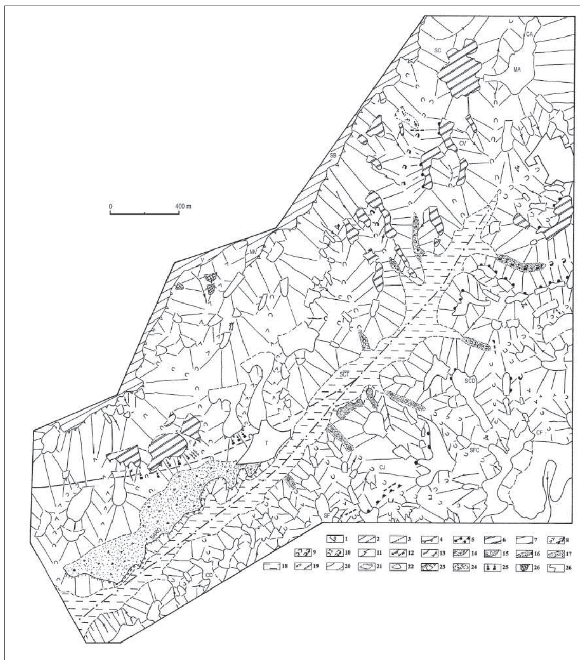
FIG. 2.6 – Mapa geomorfológico de pormenor da bacia da Ribeira de Toledo: 1 - Magnitude e sentido de inclinação das camadas; 2 : Falha certa e provável; 3: Falha deduzida; 4: Escarpa de falha degradada; 5: Rebordo de relevo monoclinal conservado ou degradado; 6: Superfície estrutural ou subestrutural; 7: Nível da Ventosa; 8: Vale de fundo em “V” simétrico e dissimétrico; 9: Vale de fundo em “U” simétrico e dissimétrico; 10: Vale de fundo plano simétrico e dissimétrico; 11: Sulcos ou ravinas; 12: Ravinamento generalizado; 13: Rebordo de terraço suave ou abrupto; 14: Elemento de terraço com cobertura coluvionar; 15: Elemento de terraço com depósito de textura fina; 16: Enchimento aluvial com material heterométrico; 17: Enchimento aluvial com material fino; 18: Planície aluvial holocénica; 19: Ruptura no declive longitudinal do curso de água; 20: Alto e base de vertente; 21: Portela; 22: Rechã; 23: Aumento localizado de declive; 24: Deslizamento provável; 25: Desabamentos; 26: Patamares antrópicos; 27: Povoações. SC: Sítio do Corvo; CA: Casais do Araújo; MA: Moinhos do Araújo; SB: Sítio das Bicas; CV: Casal do Valvito; MV: Moinhos da Ventosa; V: Ventosa; T: Toledo; SCT: Sítio da Costa; SCD: Sítio do Caldeirão; CF: Casal da Falda; SFC: Sítio da Fonte de Cima; CJ: Casais do Juncal; SF: Sítio da Formiga; CD: Casal do Delgado; CD: Casal do Delgado; SF: Sítio da Formiga; SARQ: Sítio arqueológico de Toledo.
