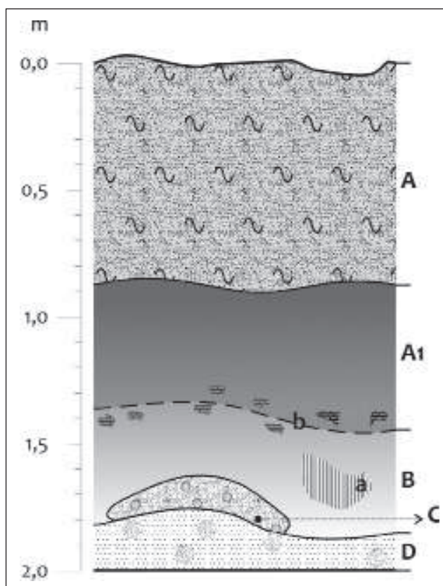
FIG. 2.7 - Variação de fácies ao longo do corte do horizonte arqueológico de Toledo. D: material arenoso fino esbranquiçado, com “bonecas” de calcário, substrato jurássico; C: areias amarelas claras com conchas inteiras e instrumentos em sílex; B: horizonte de concheiro, com estruturas de combustão (a) e com leito com grande abundância de clastos angulosos (b); A1: sedimento argilo-arenoso castanho acinzentado; A: sedimento argilo-arenoso castanho claro. A designação dos horizontes encontra-se de acordo com as referências apresentadas por Araújo (1998).
