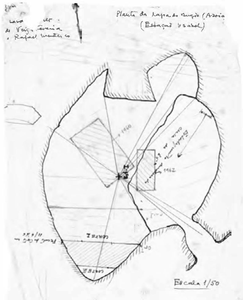
Fig. 9 – Contorno do interior da Lapa do Bugio, em papel vegetal, correspondendo ao primeiro levantamento à prancheta realizado, com a implantação das áreas escavadas até 1960, e em 1962 por Agostinho Farinha Isidoro.
