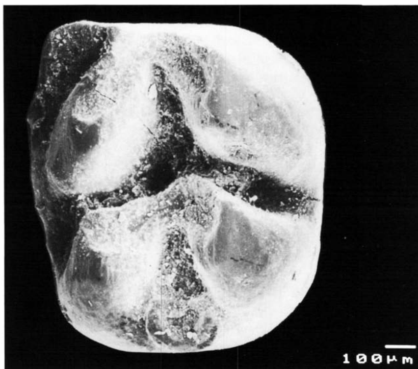
Fig. 13 – Apodemus sylvaticus . M/2 esquerdo. Foto de J. Pais ao microscópio electrónico de varrimento da FCT/UNL (Centro de Estudos Geológicos).
