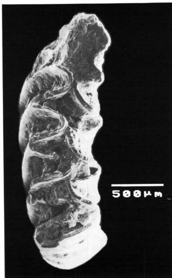
Fig. 11 – Pytymis duodecimcostatus . M/1 direito. Foto de J. Pais ao microscópio electrónico de varrimento da FCT/UNL (Centro de Estudos Geológicos).
