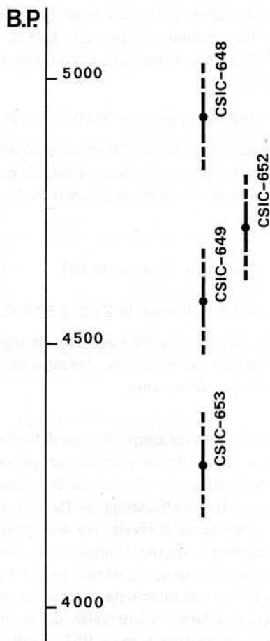
Fig. 8 — Datas convencionais de radiocarbono para o Neolítico da Comporta (intervalo de 1\sigma , representado a cheio; intervalo de 2\sigma , a tracejado).
