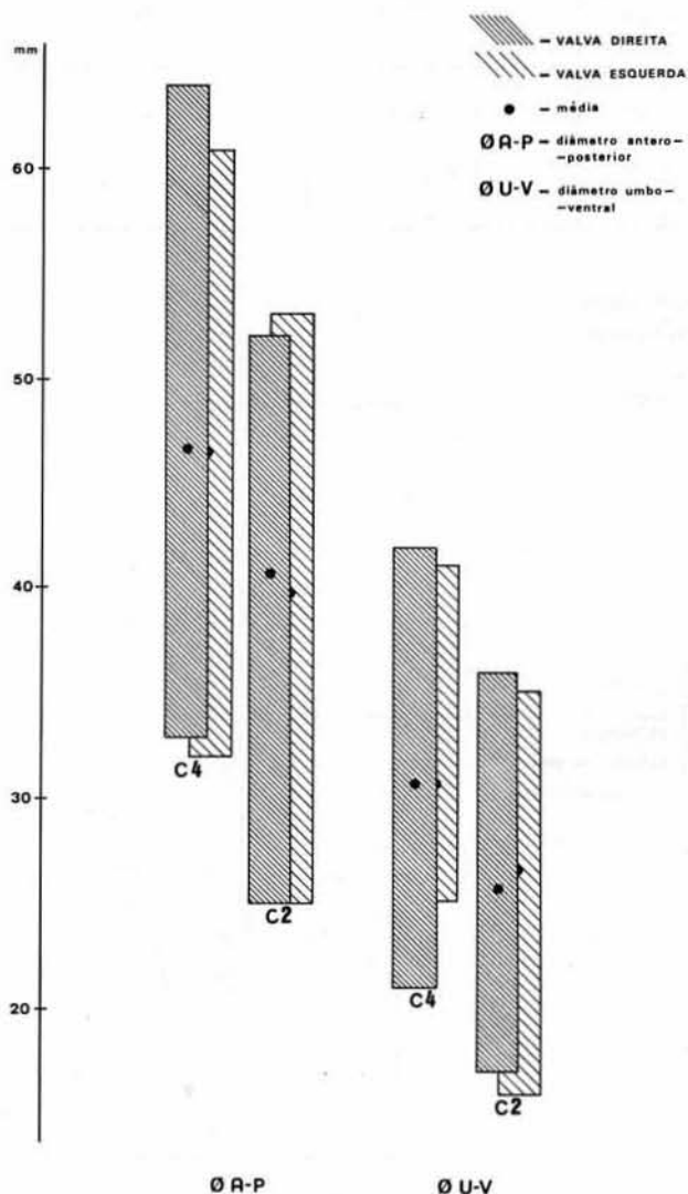
Fig. 13 — Barrosinha. Dimensões das valvas de Rudites decussatus .
