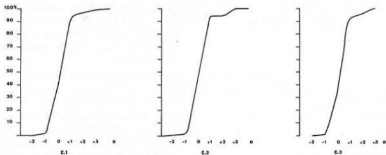
Fig. 10 — Malhada Alta — Curvas granulométricas cumulativas das camadas identificadas.
