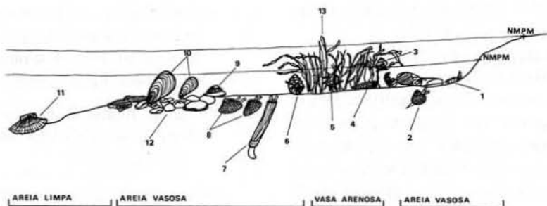
Fig. 17 — Perfil tipo da distribuição da malacofauna encontrada nas jazidas neolíticas da Comporta. 1 — Hinia reticulata ; 2 — Cerastoderma edule ; 3 — Monodonta sp.; 4 — Cerithium vulgatum ; 5 — Murex sp.; 6 — Thais haemastoma ; 7 — Solen marginatus ; 8 — Ruditapes decussatus ; 9 — Balanus sp.; 10 — Mytilus sp.; 11 — Pecten maximus ; 12 — Conchas/pedras; 13 — Gramíneas ( Zoostera sp.).
