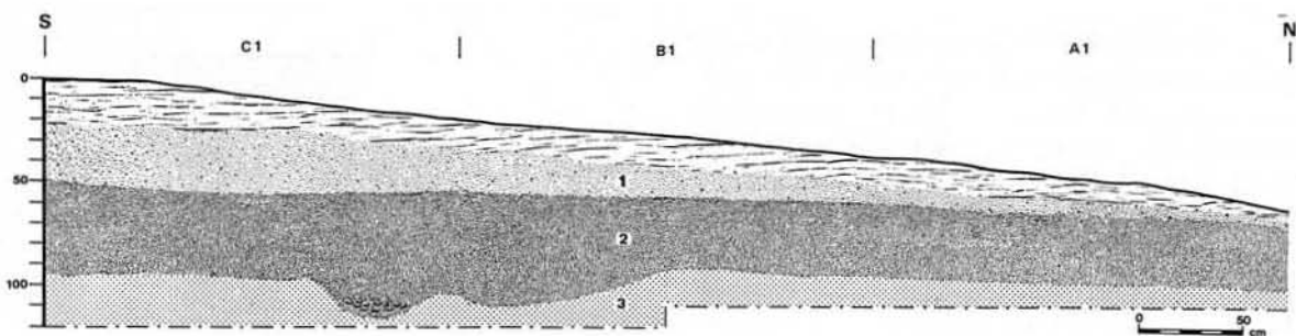
Fig. 4 — Pontal (Comporta I). Perfil Oeste dos Qs. A1-C1.
