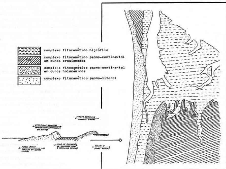
Fig. 11 — Macrozonagem vegetal da zona da Comporta.
