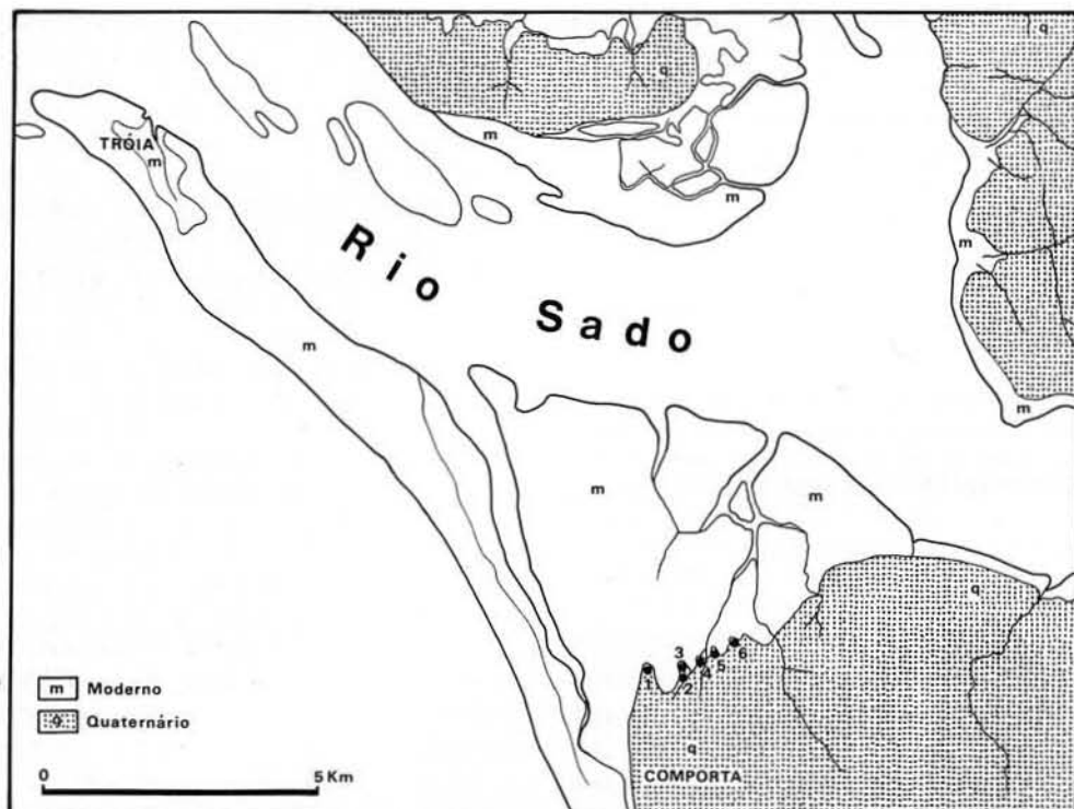
Fig. 1 — Localização das jazidas neolíticas da Comporta. Foi utilizada a carta geológica levantada por Carlos Ribeiro (Comissão Geológica, 1867). 1 — Celeiro Velho; 2 — Possanco; 3 — Malhada Alta; 4 — Pontal; 5 — Barrosinha; 6 — Sapalinho.
