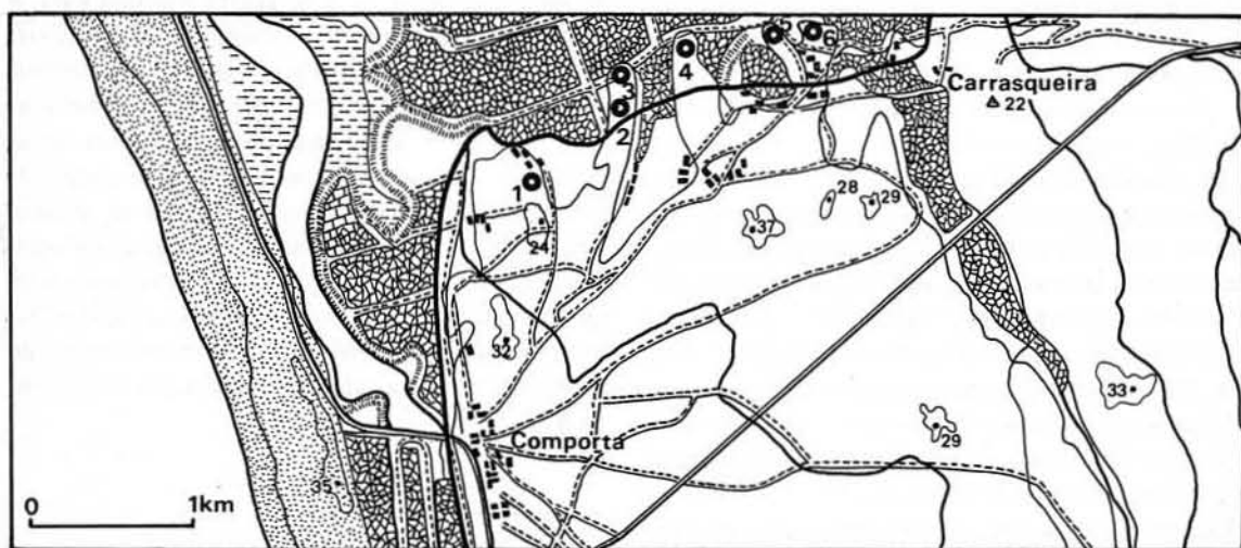
Fig. 2 — Localização das jazidas neolíticas da Comporta na carta de esc. 1:50 000. 1 — Celeiro Velho; 2 — Possanco; 3 — Malhada Alta; 4 — Pontal; 5 — Barrosinha; 6 — Sapalinho.
