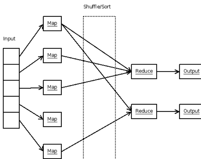
Figura 3 - Fluxo do processo MapReduce
