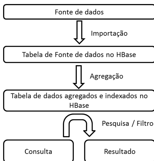
Figura 4 - Processo desde a fonte de dados até ao resultado da agregação
