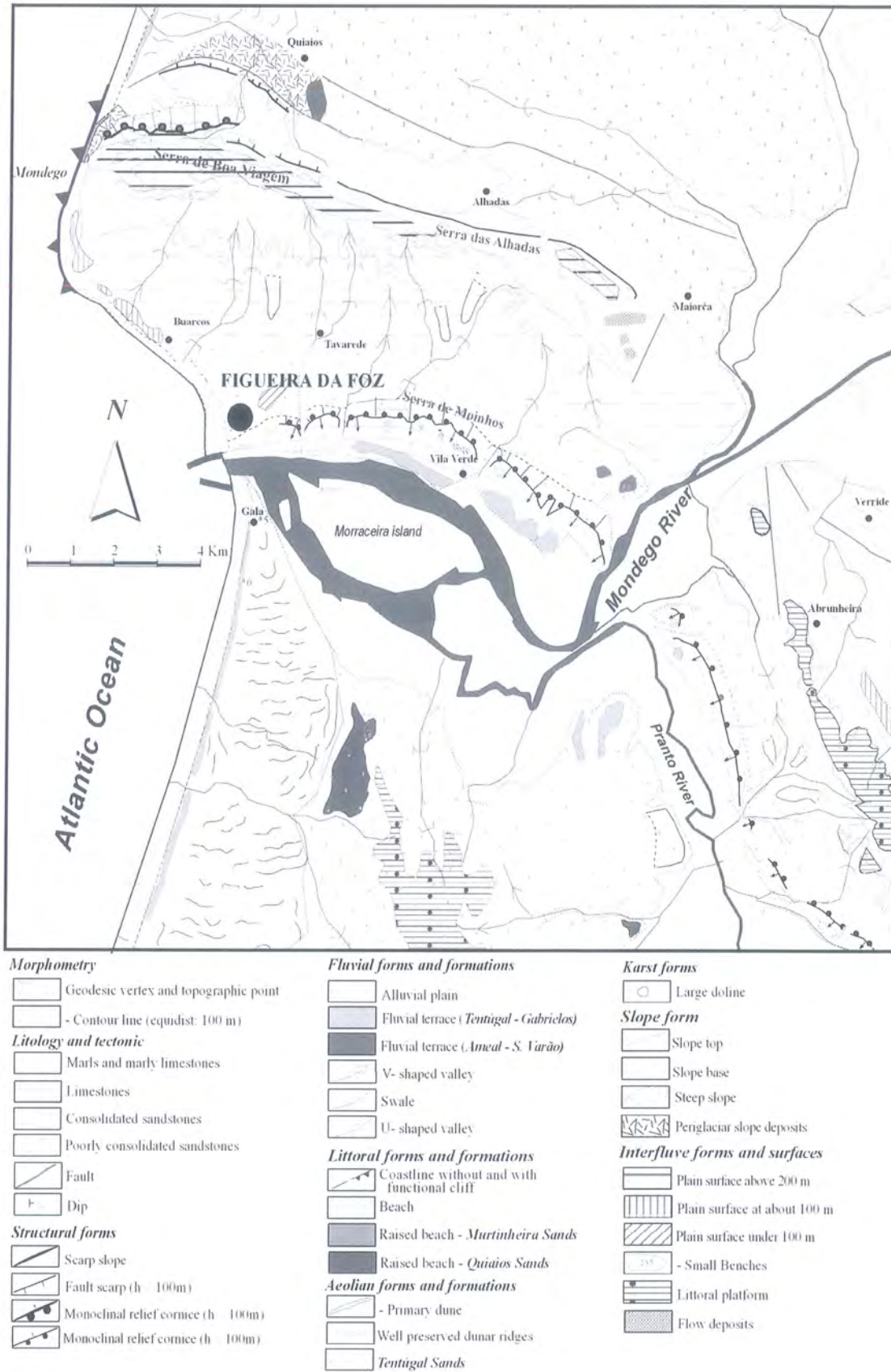
Fig. 5.1 – Geomorphological map of the Figueira da Foz region. (A. Ramos & L. Cunha).
