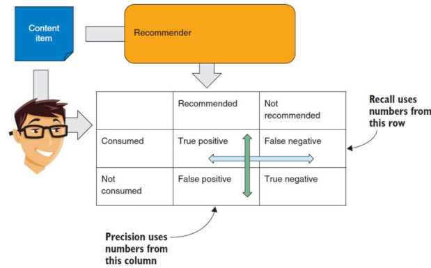
Figura 8. Formação do cálculo utilizado nas métricas precision (por colunas) e recall (por linhas) na relação entre itens recomendados e consumidos/visitados, retirada de Falk [2019, p. 226].
