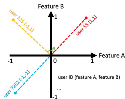
Figura 6. Exemplo de um embedding vetorial bidimensional.
