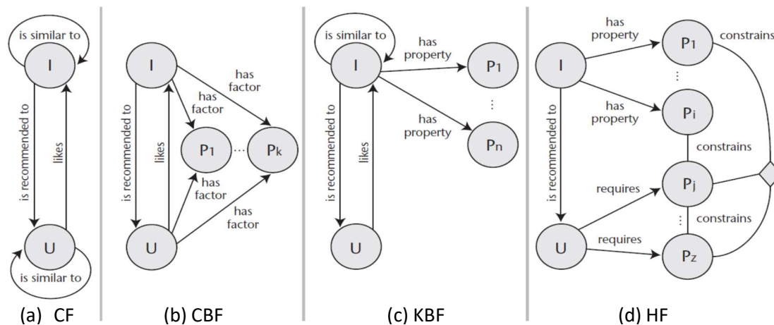
Figura 5. Arquétipos dos sistemas de recomendação, retirados de Friedrich e Zanker [2011].
